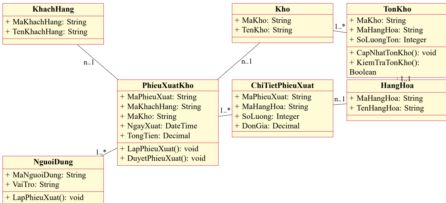
Hình 1: Biểu đồ lớp trong ca sử dụng UC10 – Lập phiếu xuất kho
